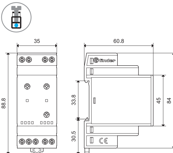
11.42 Винтовой зажим
